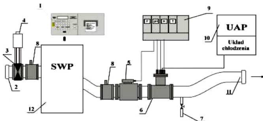
Schemat stacji zlewnej [1]: 1 – panel sterujący komputerem, 2 – złącze typu strażackiego, 3 – zasuwa nożowa \dot{C} 125, 4 – siłownik pneumatyczny, 5 – przepływomierz Dn 125, 6 – kolektor pomiarowy, 7 – zawór spustowy, 8 – kolektor płuczący, 9 – panel pomiarowy, 10 – układ automatycznego próbkowania, 11 – rura wylotowa, 12 – sito z prasą do skratek
